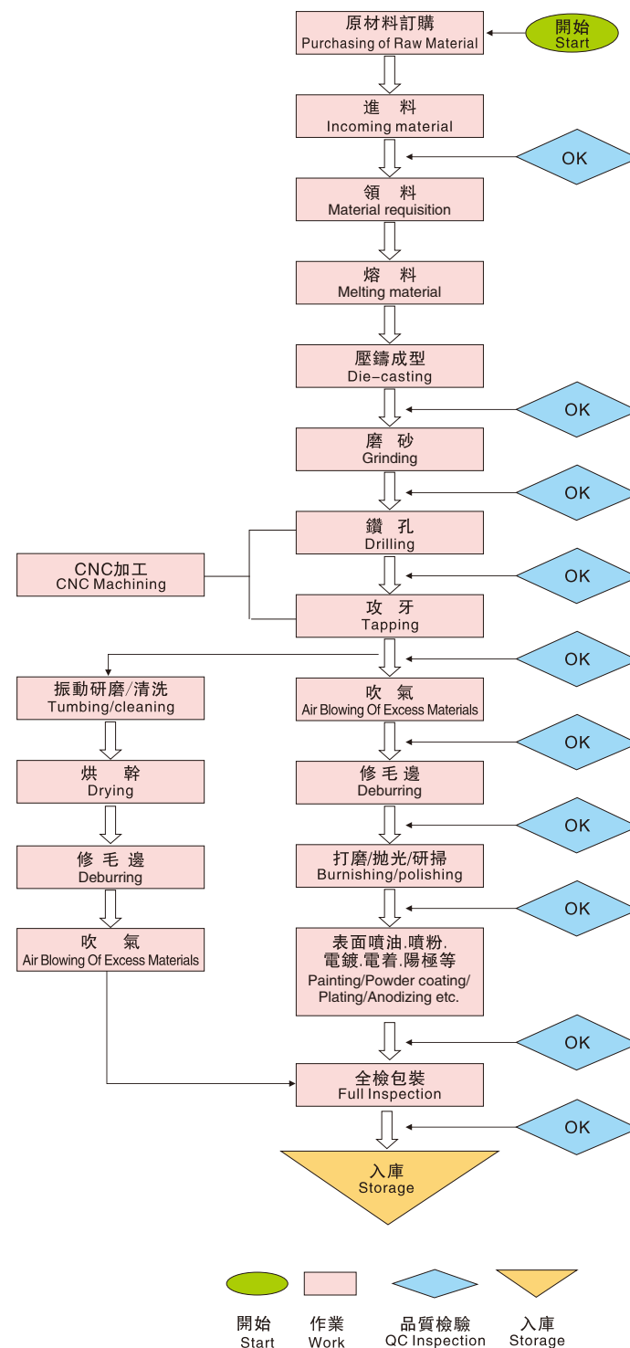
生產工藝流程圖 Process Flow Chart
